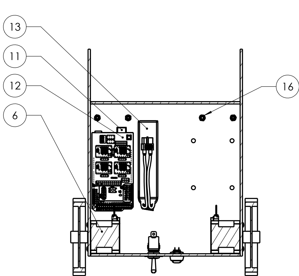
SECTION A-A
